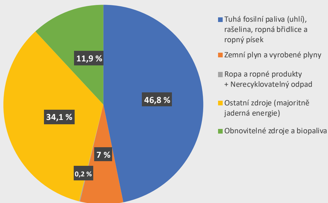
Graf 13: Hrubá výroba elektřiny v ČR v roce 2018 dle zdroje
